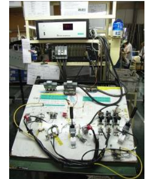
小型回路ハーネス
