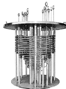
コイル式熱交換器
